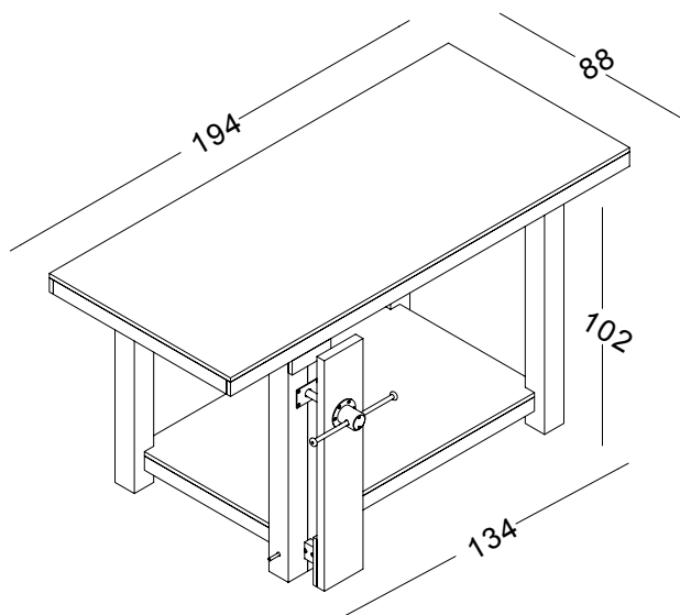
BBM dim. 194 x 88 x h102 cm banco marangon L194 cm con morsa in ferro
