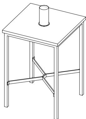
BTAf dim. 80x80xh112cm tavolo quadrato a quattro gambe con biocandela centrale 4 legs square table high with central biocandle
