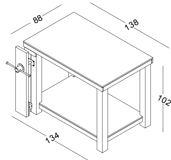
BBMP dim. 138 x 88 x h102 cm banco marangon L138 cm con morsa in ferro
