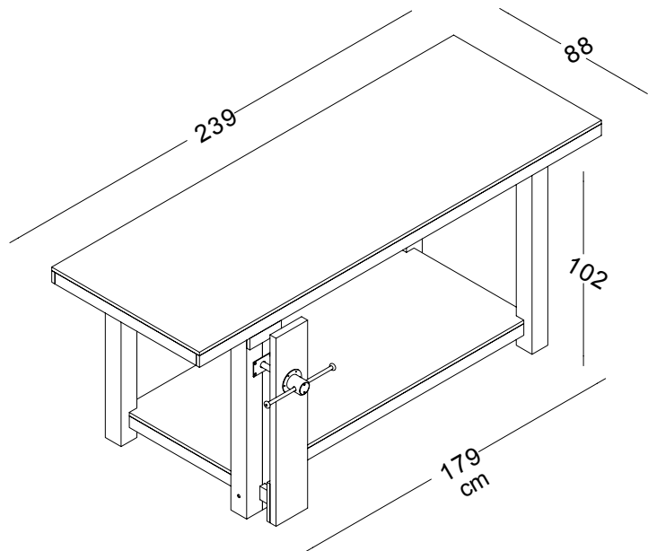
BBMG dim. 239 x 88 x h102 cm banco marangon L239 cm con morsa in ferro
